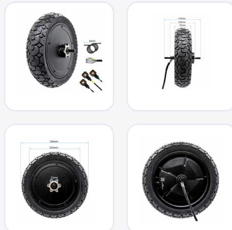
Motoransichten und Abmessungen
