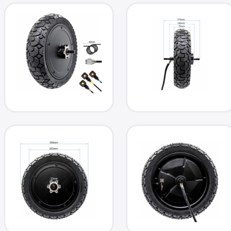
Viste del motore e dimensioni
