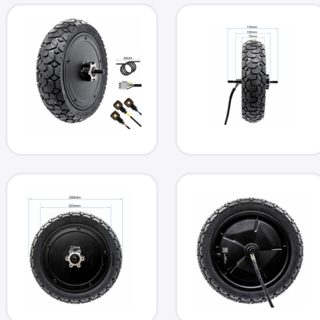
Vues du moteur et dimensions
